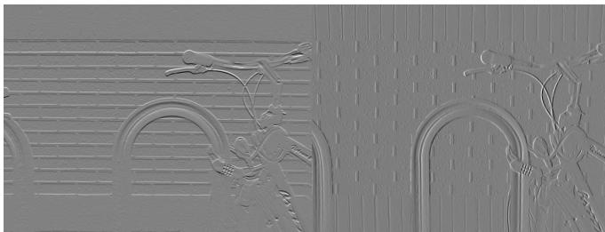
Y-gradient
