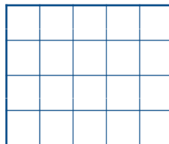
Parameter Space
